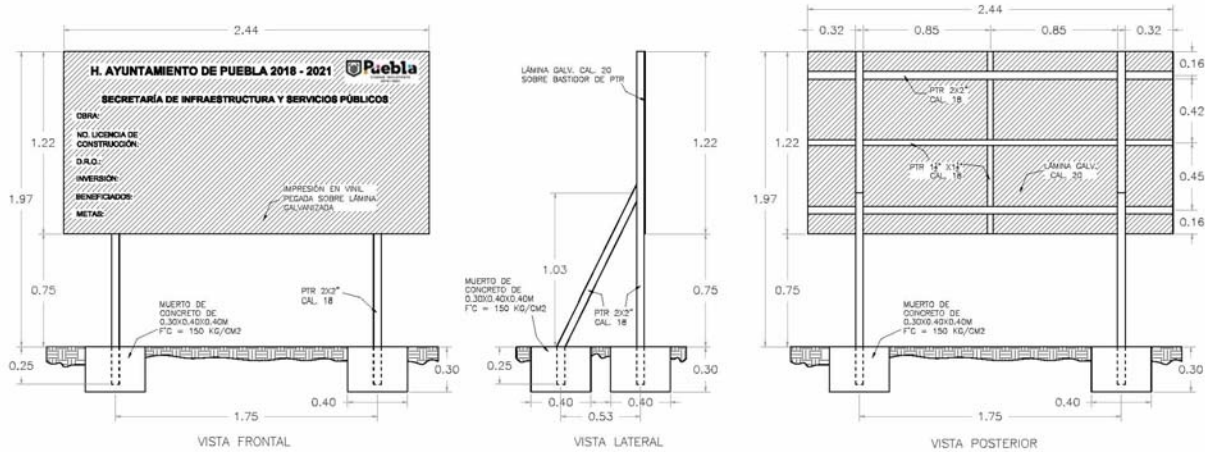
LETRERO INFORMATIVO PARA OBRAS PÚBLICAS TIPO "II"
