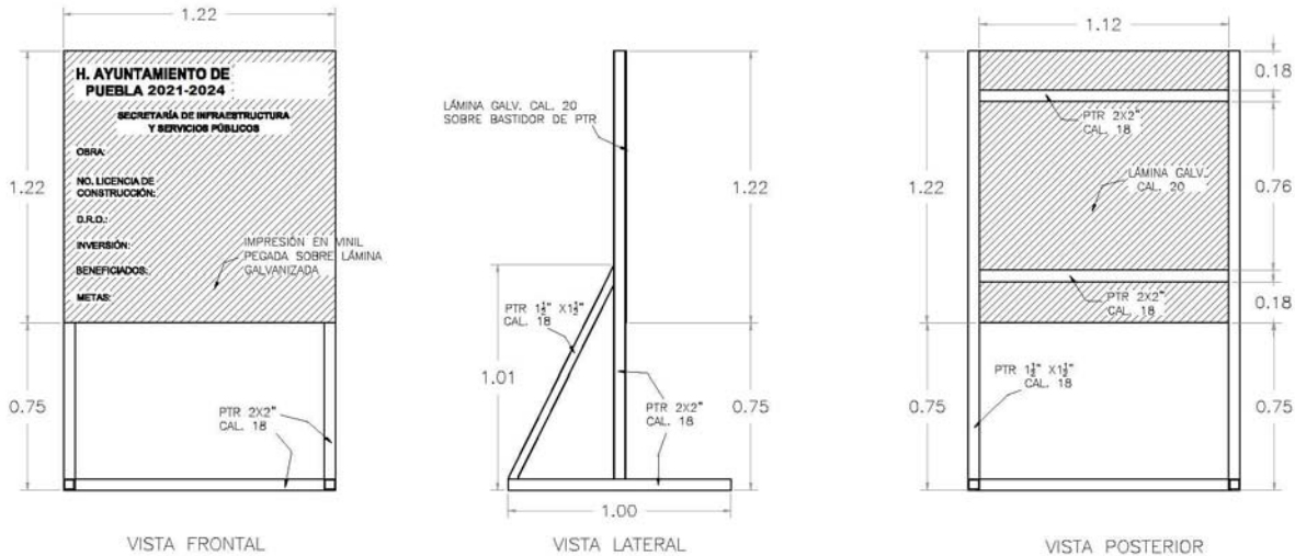
LETRERO INFORMATIVO PARA OBRAS PÚBLICAS TIPO "III"
